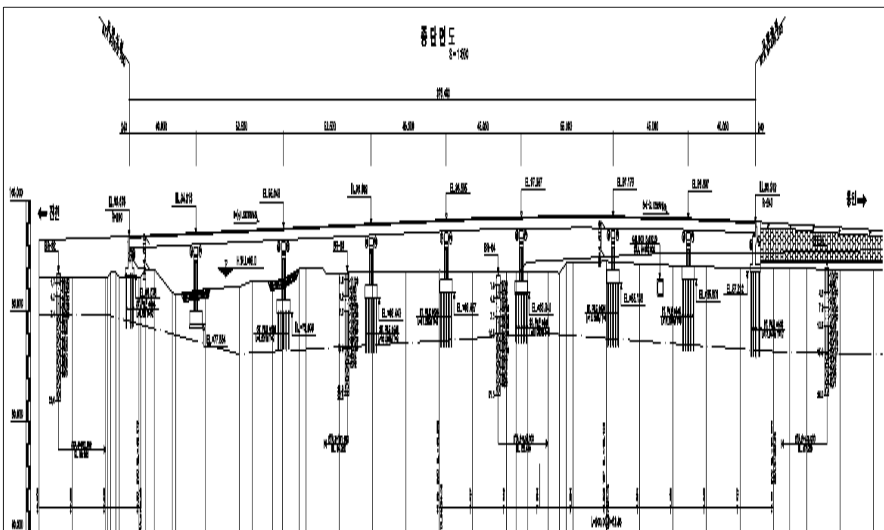
【그림 3.1.2】 축산1교(상행_용인방향) 종단면도
