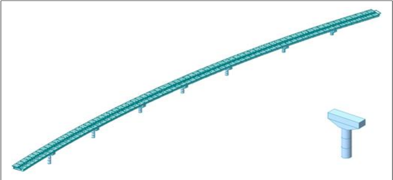
【그림 3.4.1】 축산1교(상행_용인방향) 교량 구조해석 모델링
